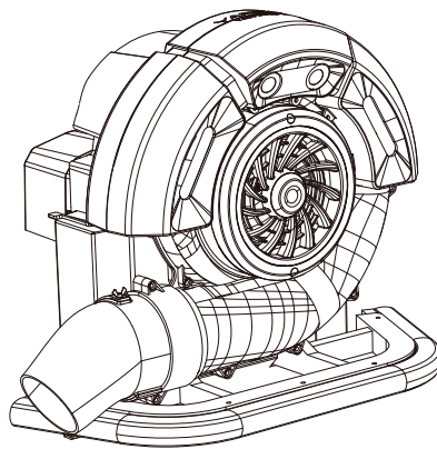
Blower Module
